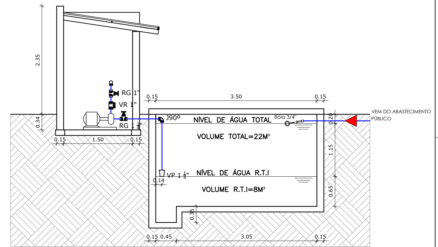
DETALHE - SUGESTÃO SISTEMA DE RECALQUE ESCALA 1:50
