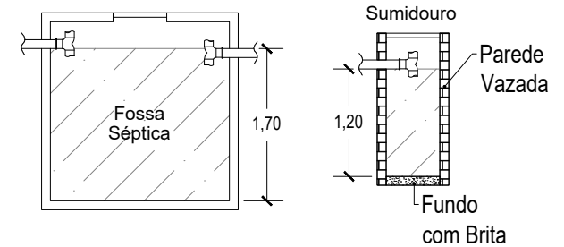
VISTA DO CORTE DA FOSSA E SUMIDOURO
