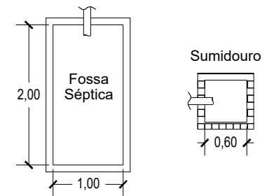
VISTA EM PLANTA DA FOSSA E SUMIDOURO
