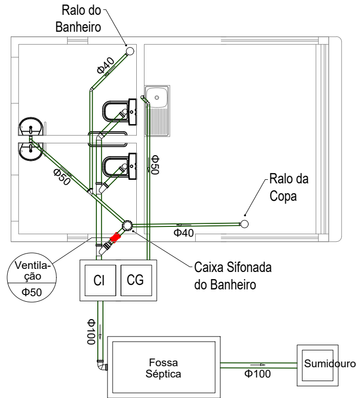
PLANTA BAIXA - ESCALA 1:75
