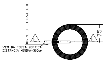
PLANTA BAIXA SUMIDOURO
