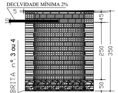
CORTE EE SUMIDOURO
