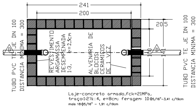
PLANTA BAIXA-TANQUE SÉPTICO
